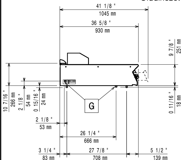
Oldalnézet
